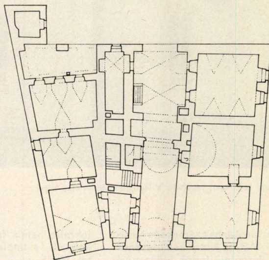
Földszinti alaprajz
