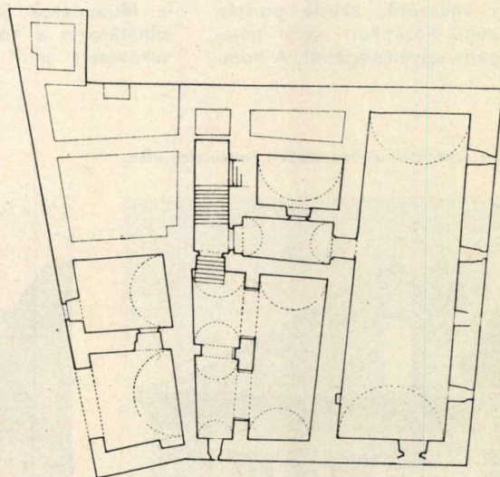
Alagsori alaprajz
